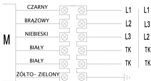
SCHEMAT ELEKTRYCZNY SILNIKA TRÓJ-FAZOWEGO
